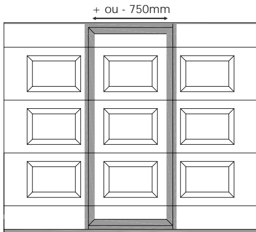
SCHEMA DE FABRICATION POUR LES PORTES CASSETTES INFÉRIEURES A 2150 DE HAUTEUR
